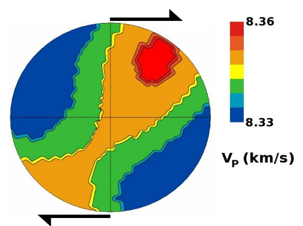
Anisotropie
