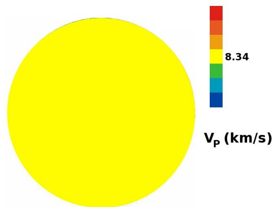
Pas d'anisotropie
