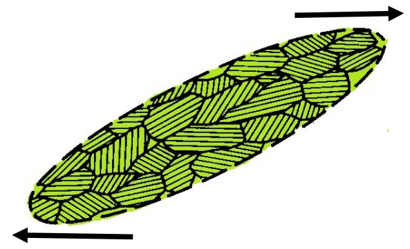
Polycristal déformé
