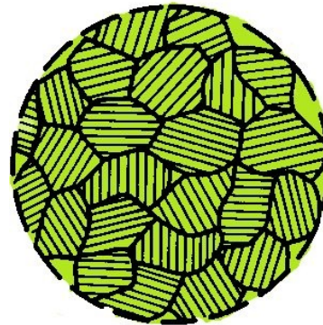
Polycristal aléatoire
